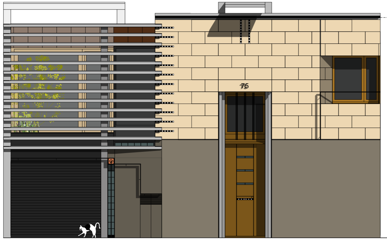
Élévation Nord
