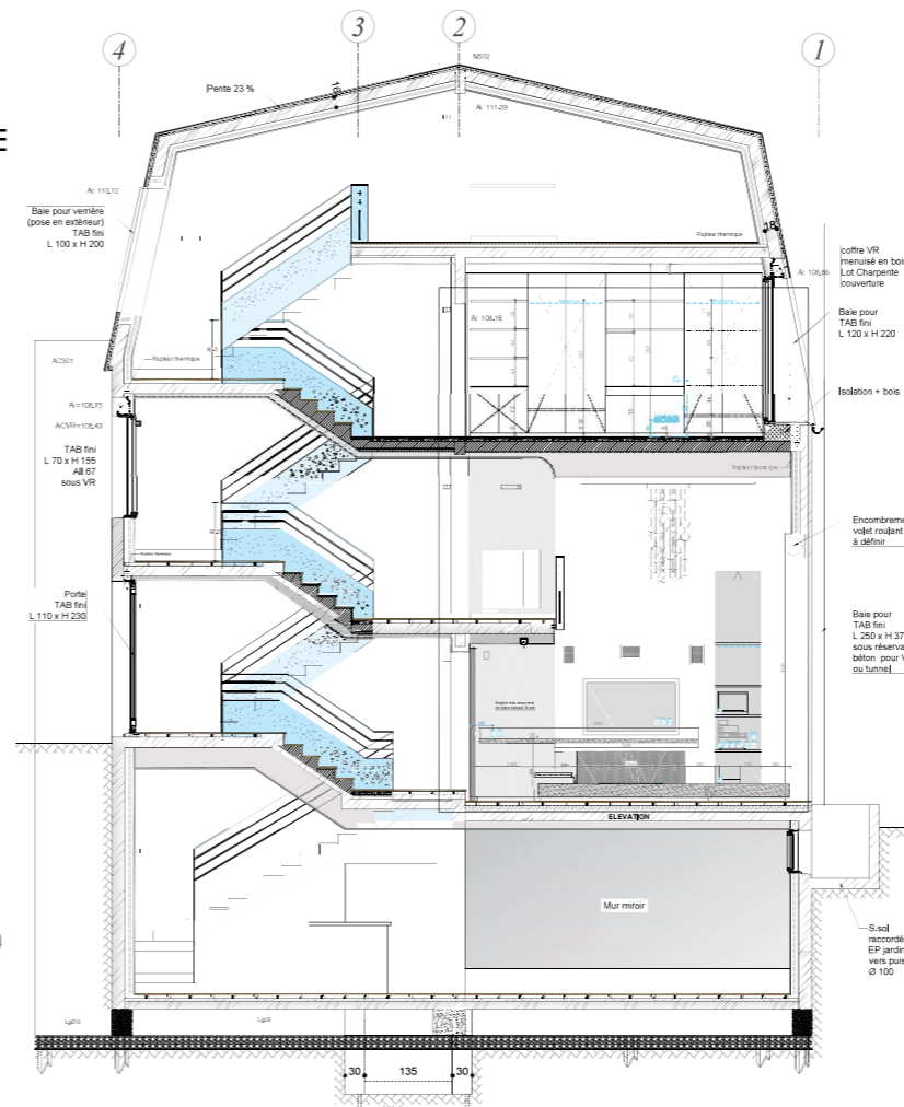
COUPE LONGITUDINALE
