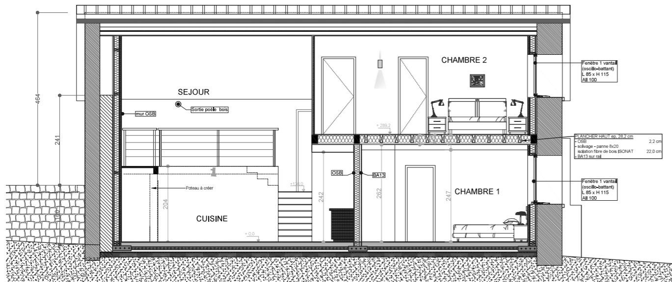
COUPE LONGITUDINALE
