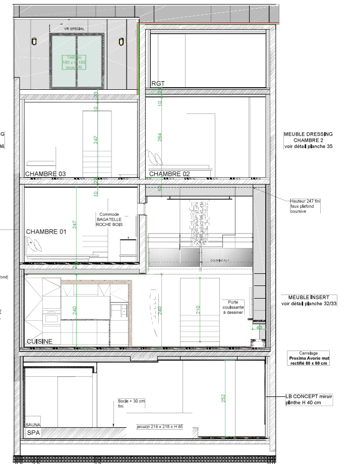
COUPE TRANSVERSALE
