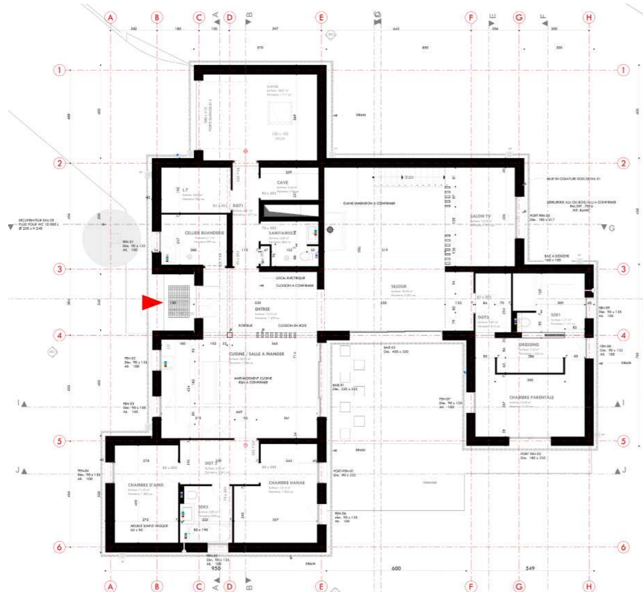
PLAN REZ DE CHAUSSEE
