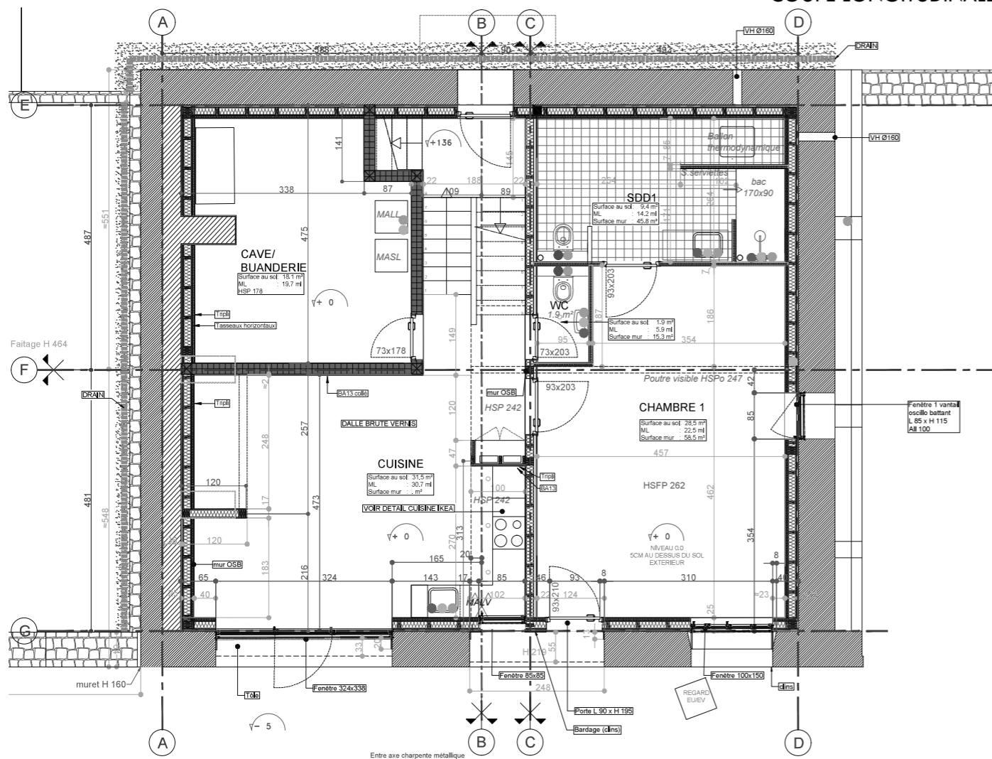
PLAN REZ DE CHAUSSEE PLATRIERIE
