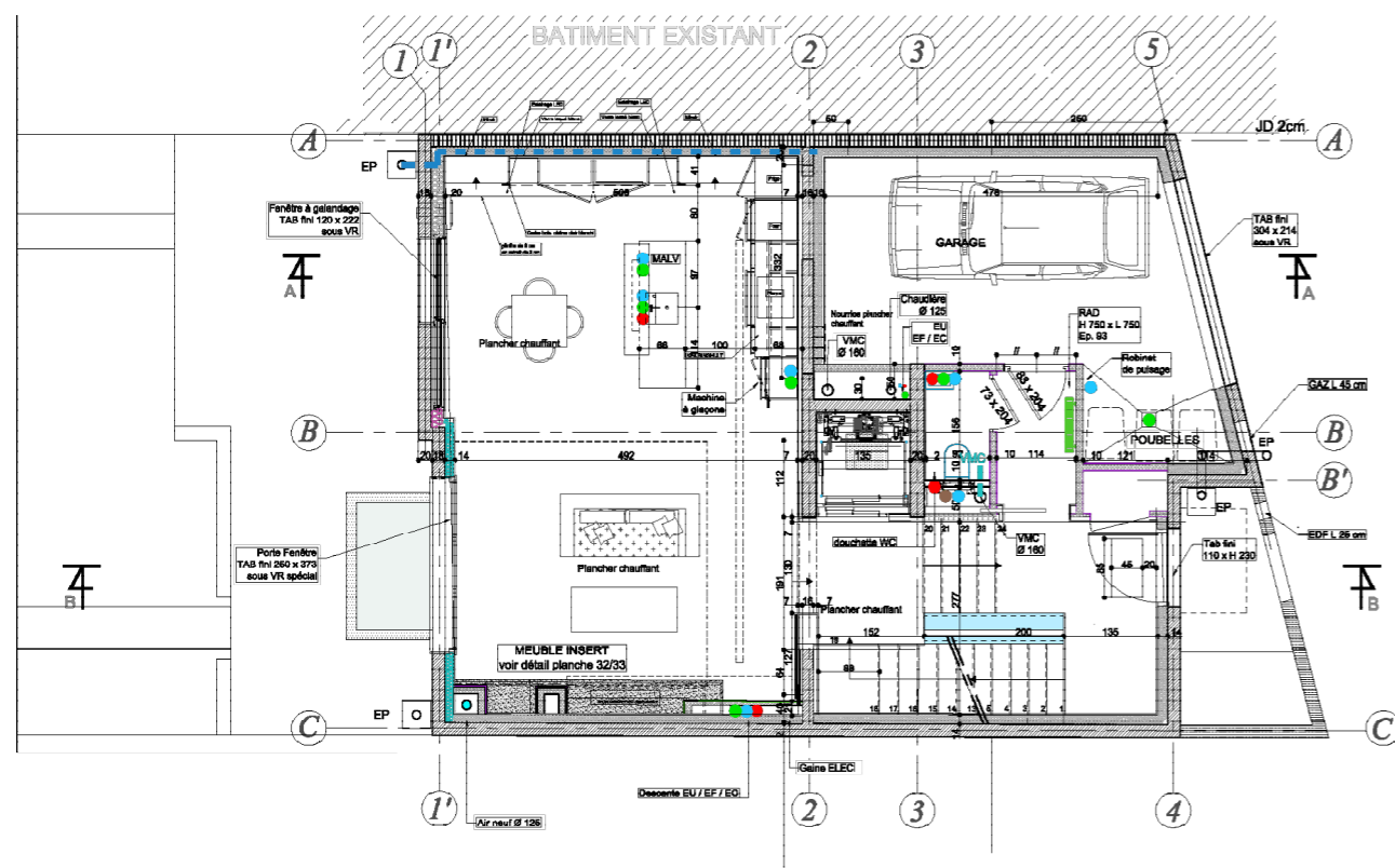
PLAN REZ DE CHUSSEE PLATRERIE
