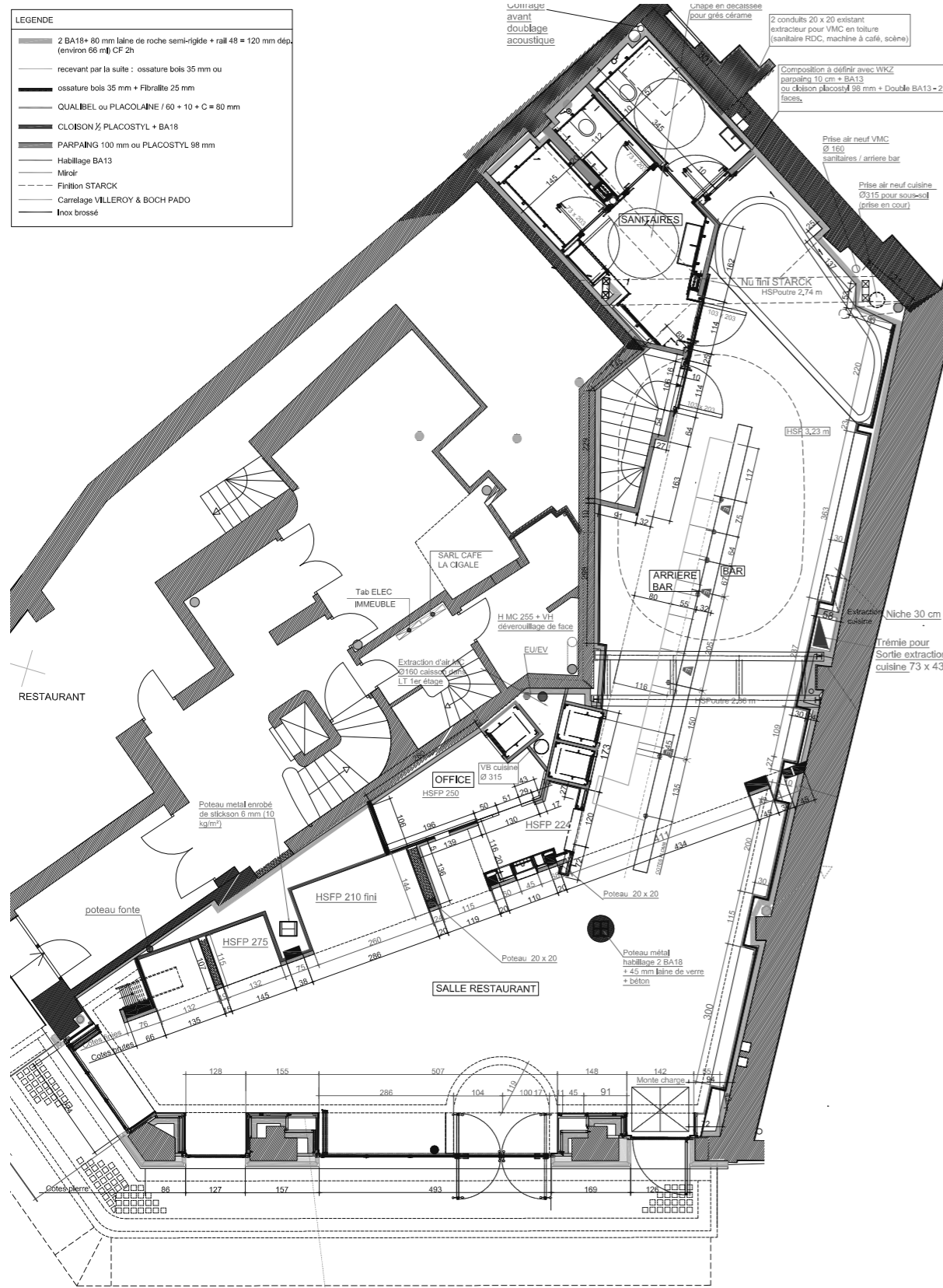
PLAN REZ DE CHAUSSEE PLATRERIE
