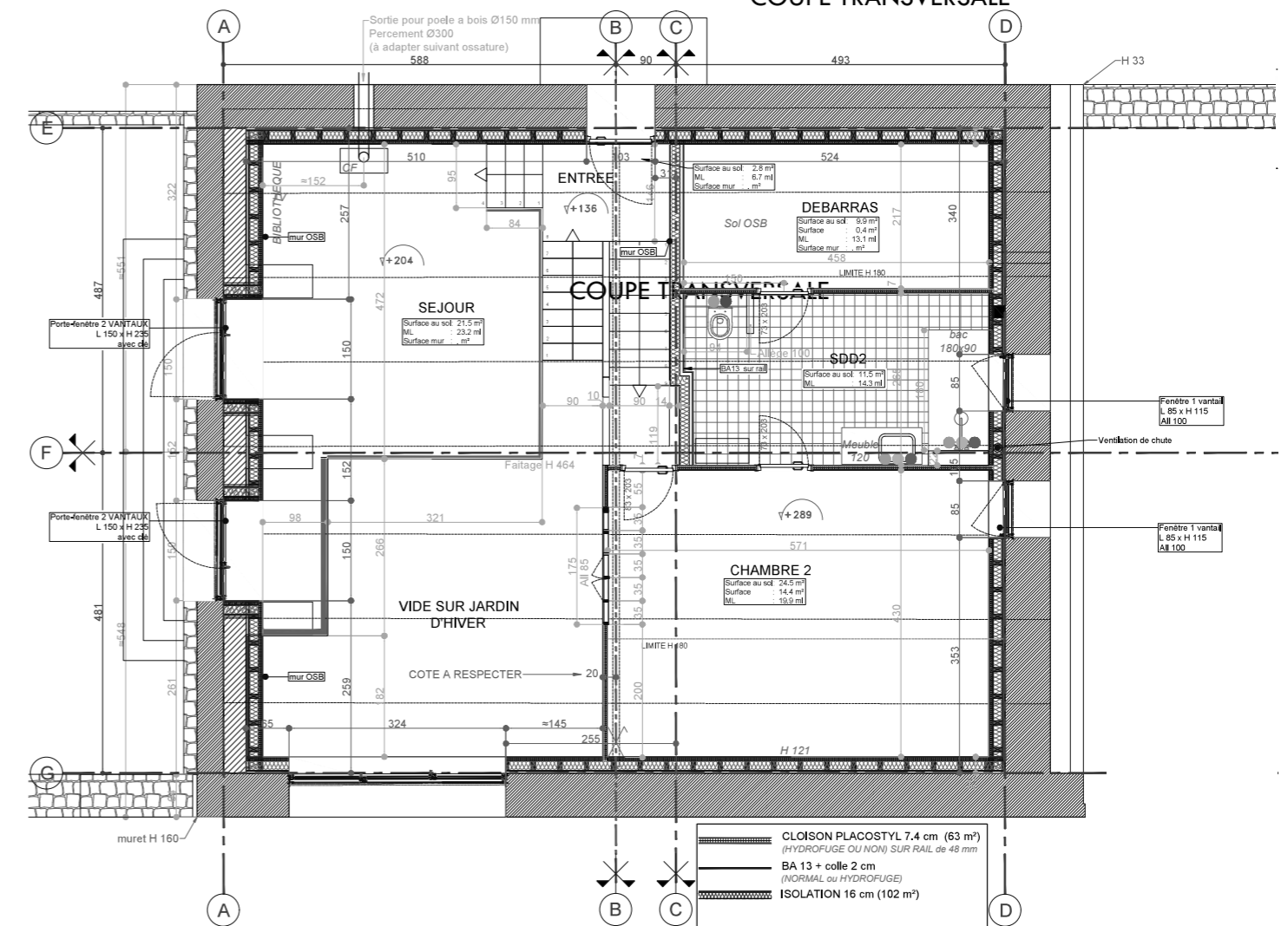
PLAN 1ER ETAGE PLATRIERIE
