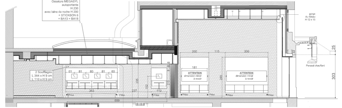
COUPE LONGITUDINALE
