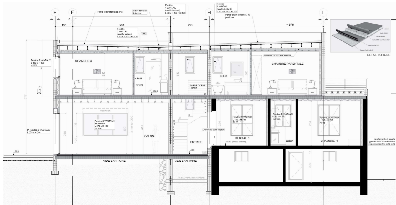
COUPE LONGITUDINALE
