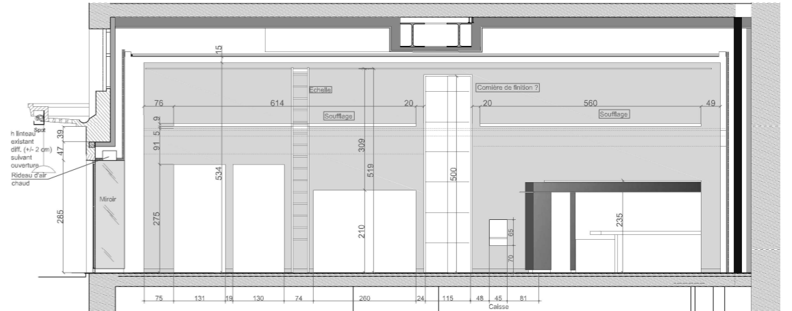
COUPE TRANSVERSALE
