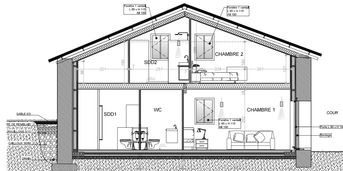
COUPE TRANSVERSALE
