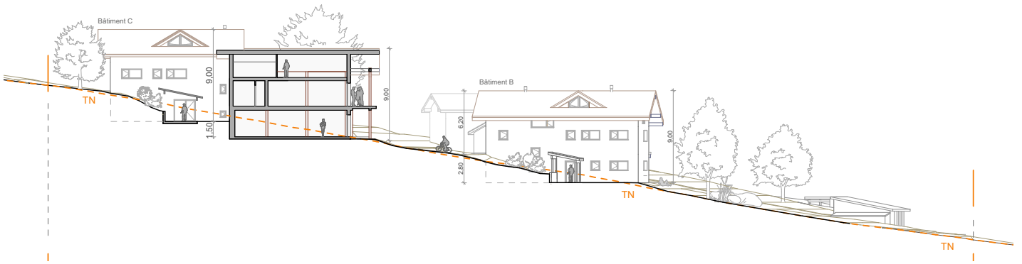
Coupe transversale : des bâtiments enchassés dans la pente, bien orientés
