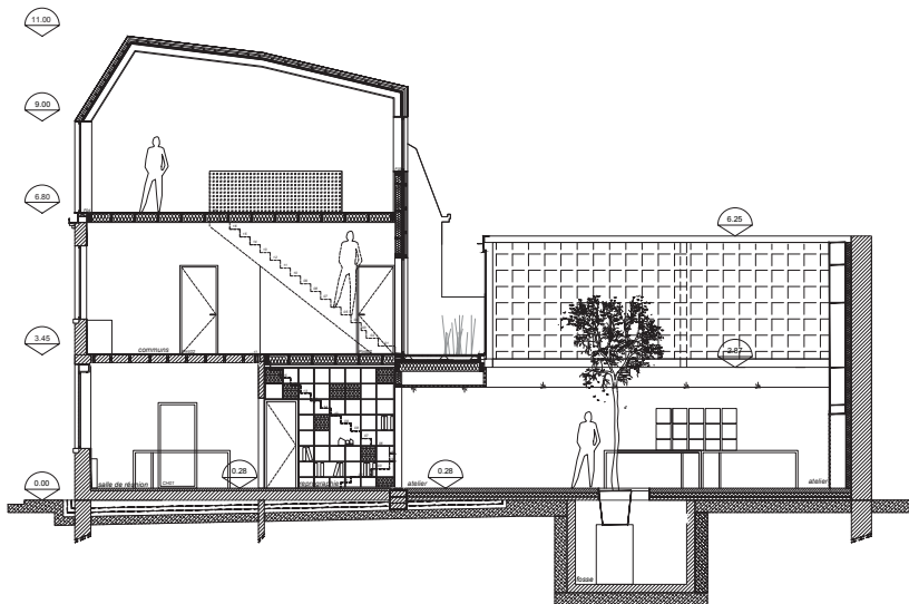
Coupe transversale
