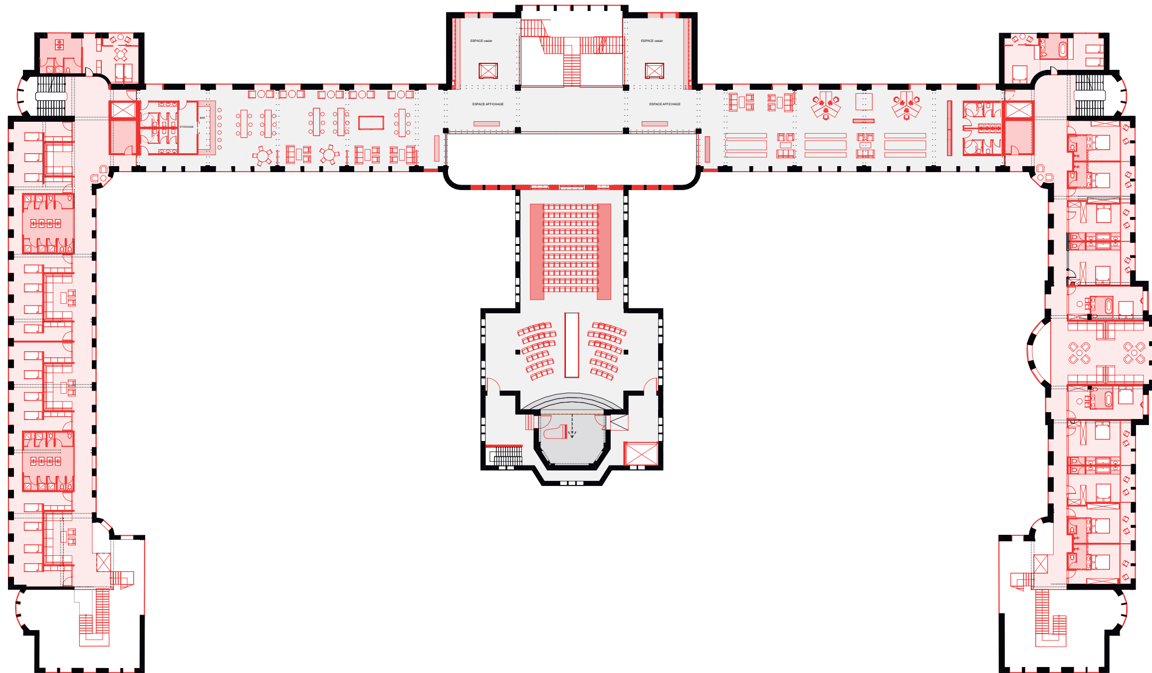
R+2 du projet
