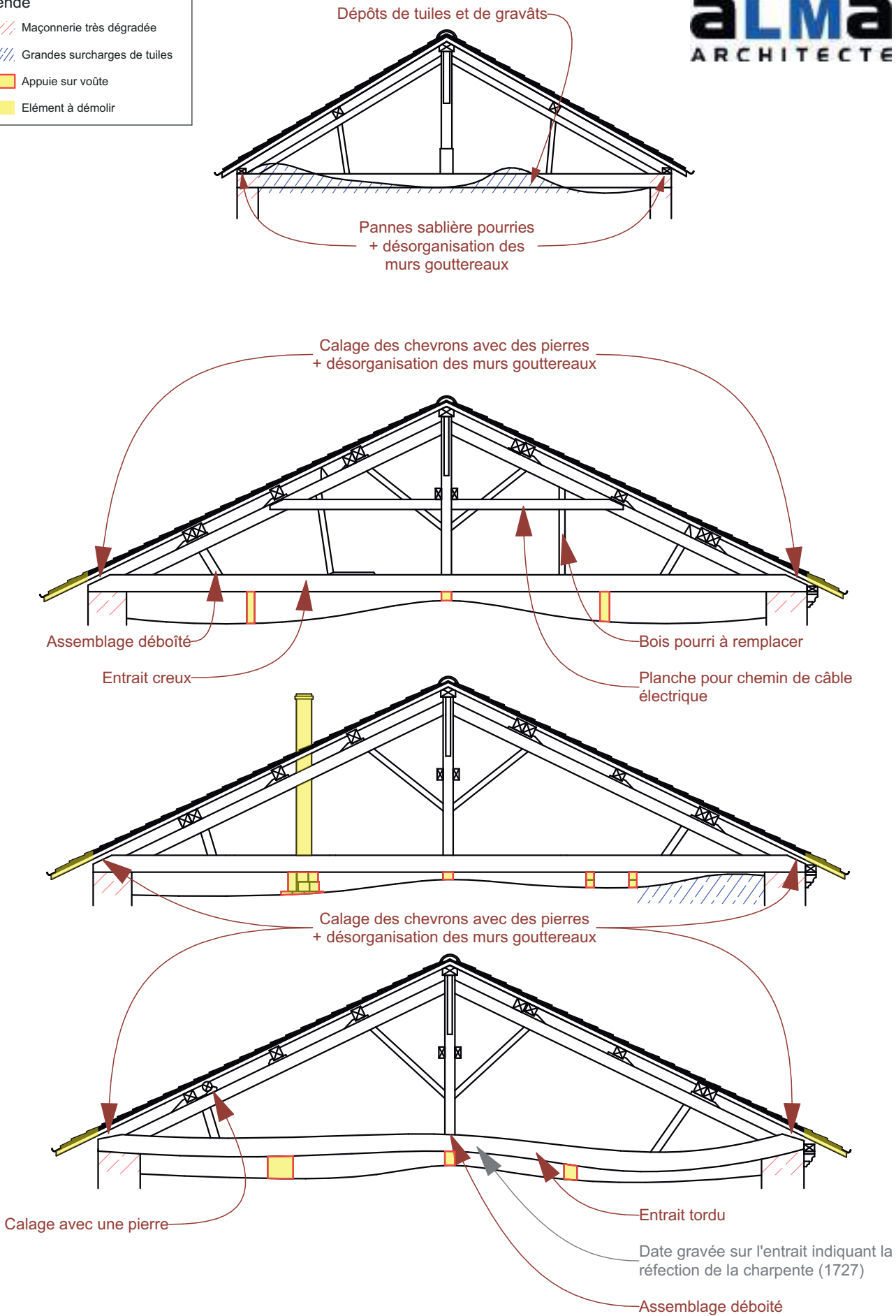
Élévation des fermes de la charpente (diagnostic)
