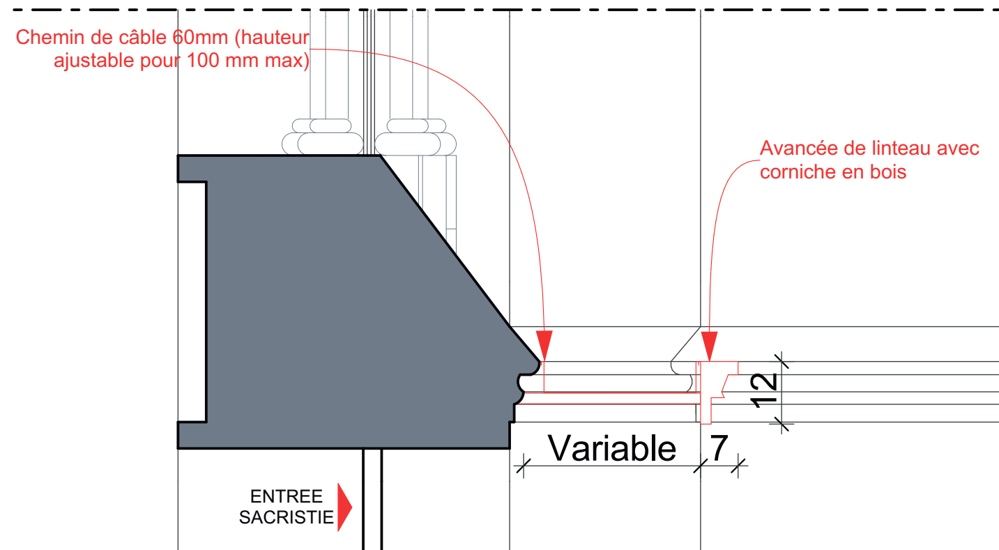
Détail du linteau à crée (projet de restauration)
