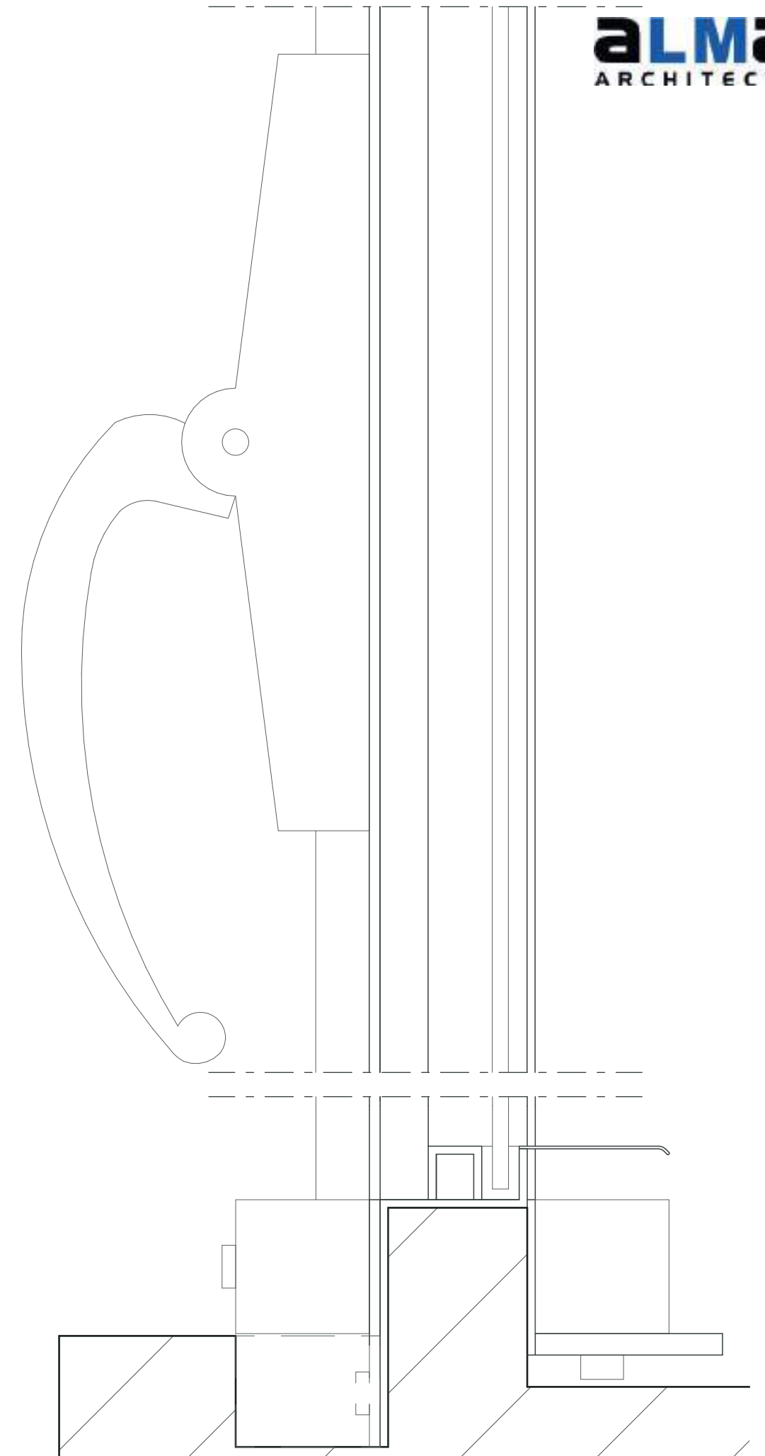
Détails des menuiseries de l'ensemble vitré en coupe (éch : 1/1)
