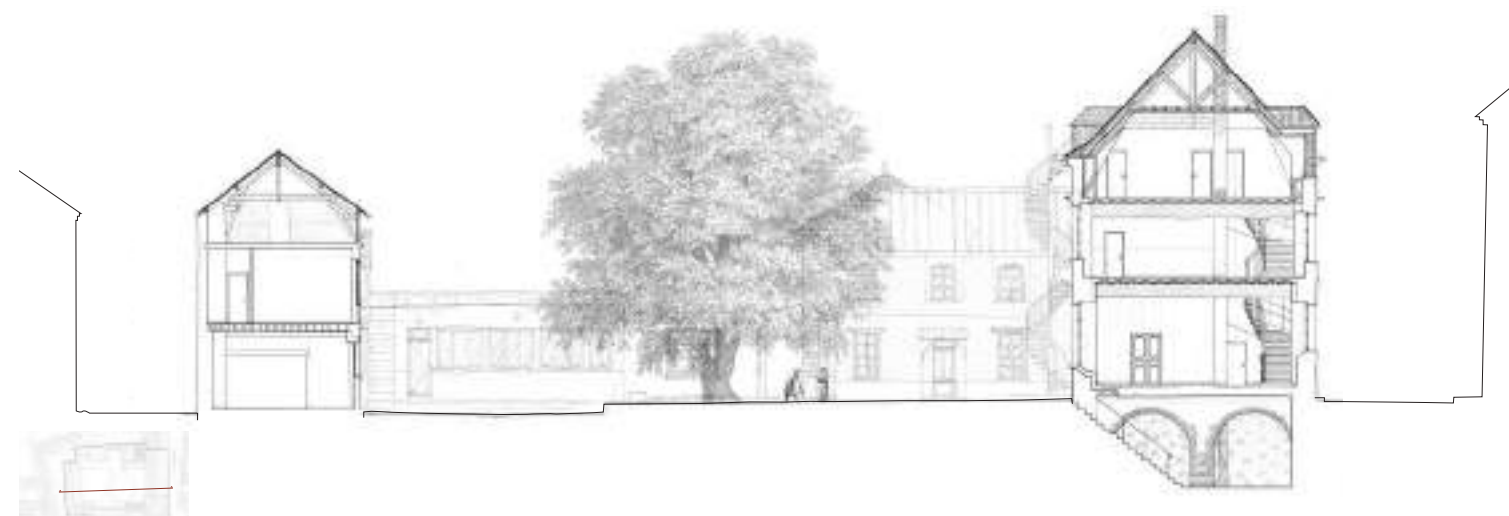
Coupe-élévation longitudinale - état existant
