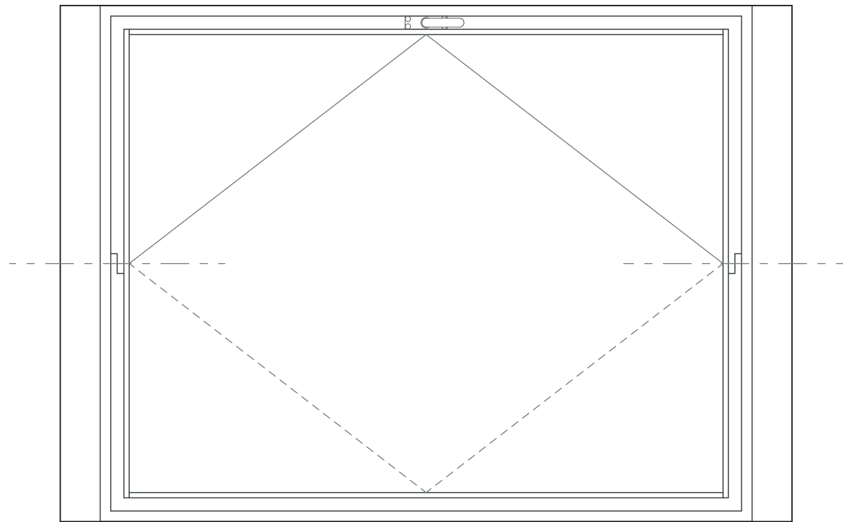
Élévation de la fenêtre de la sacristie (ech : 1/10)
