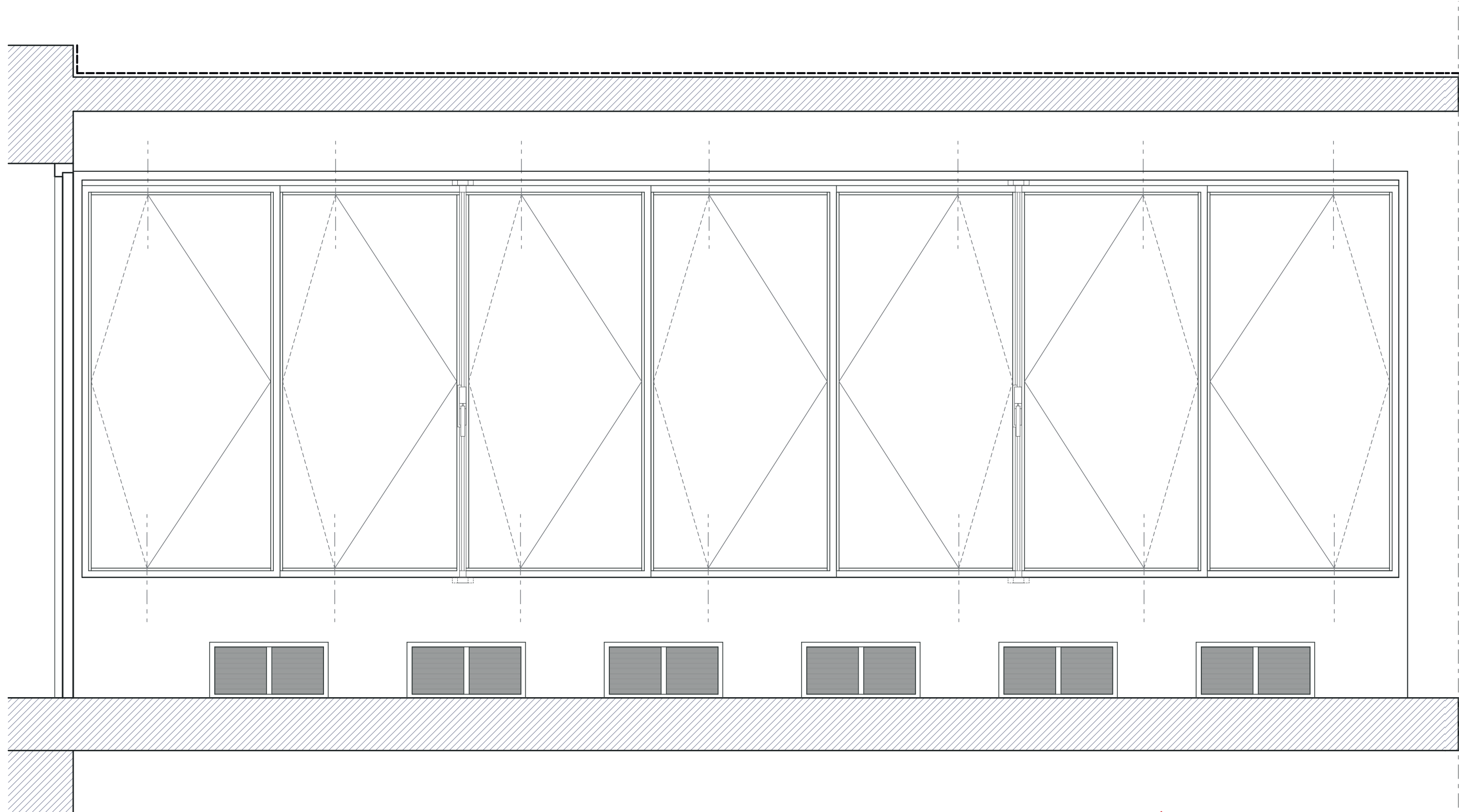
Élévation intérieure de l'ensemble vitré (éch : 1/15)
