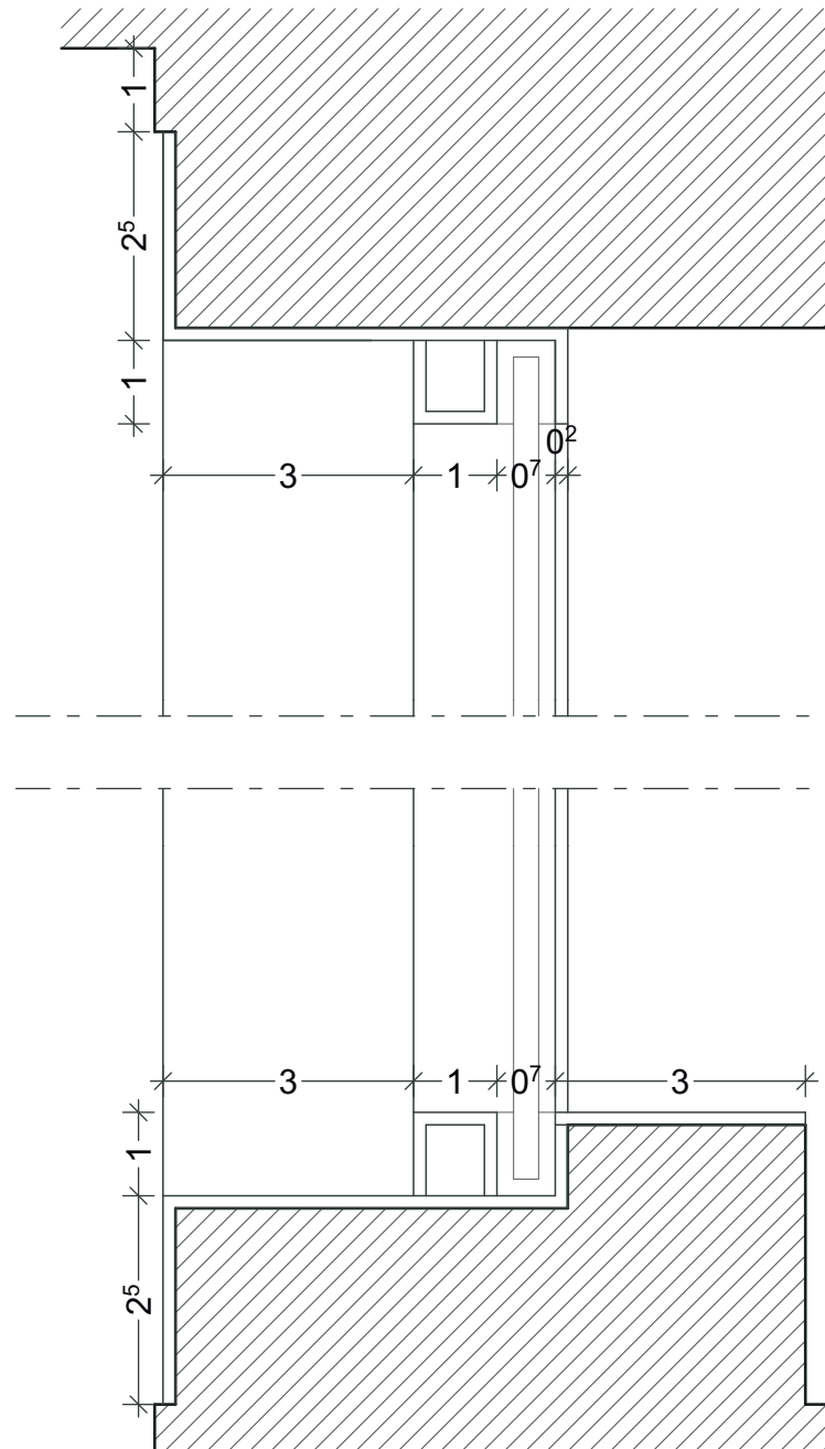
Détail du châssis fixe en élévation (éch : 1/1)
