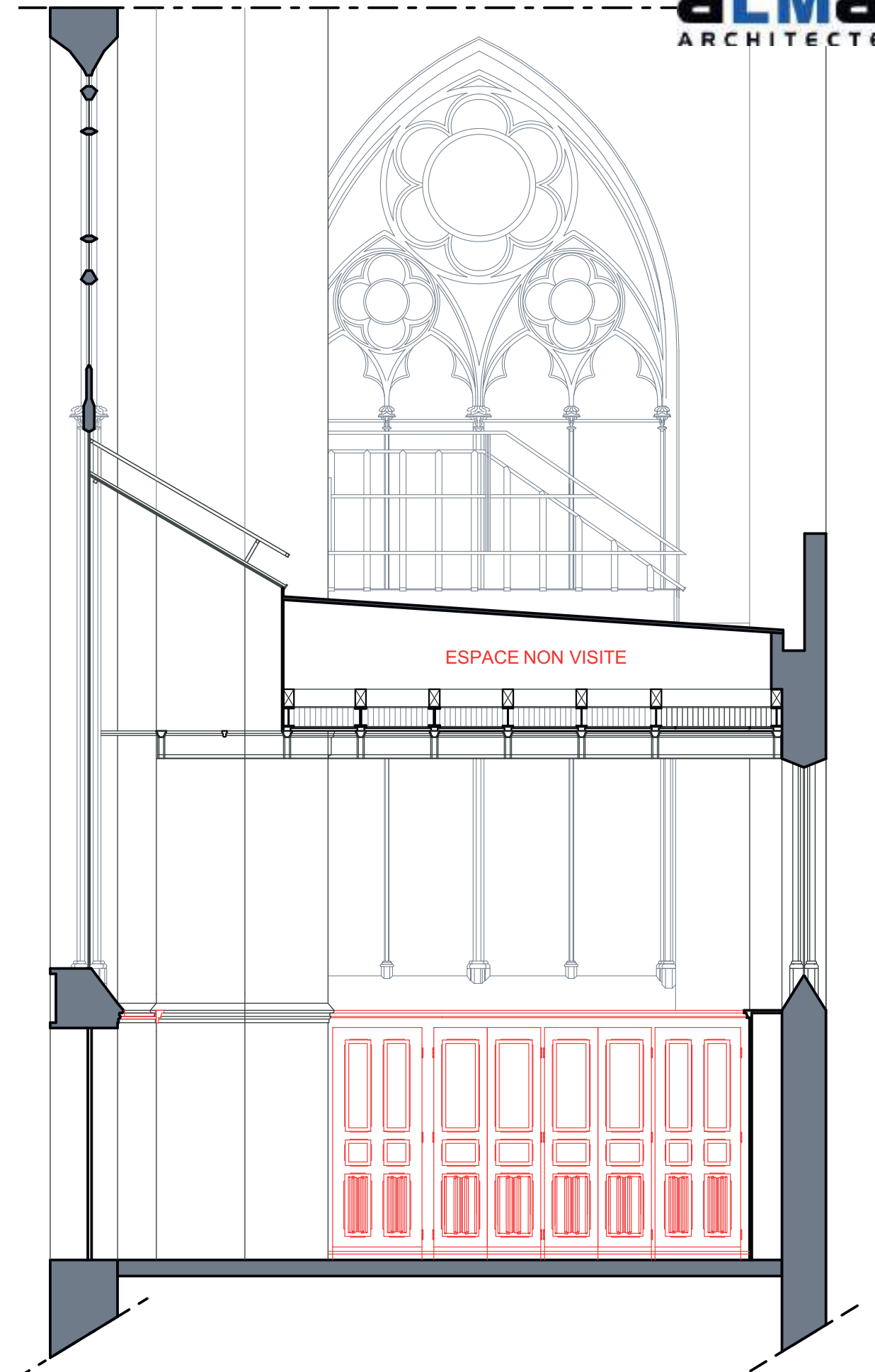
Élévation intérieure nord (projet de restauration)
