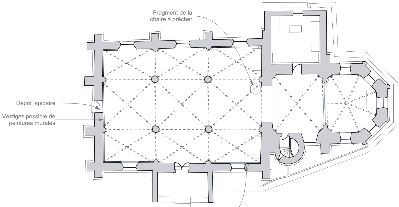
Plan RDC
