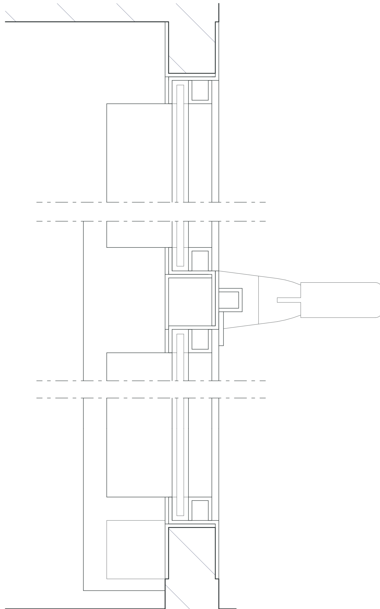
Détails des menuiseries de l'ensemble vitré en plan (éch : 1/1)
