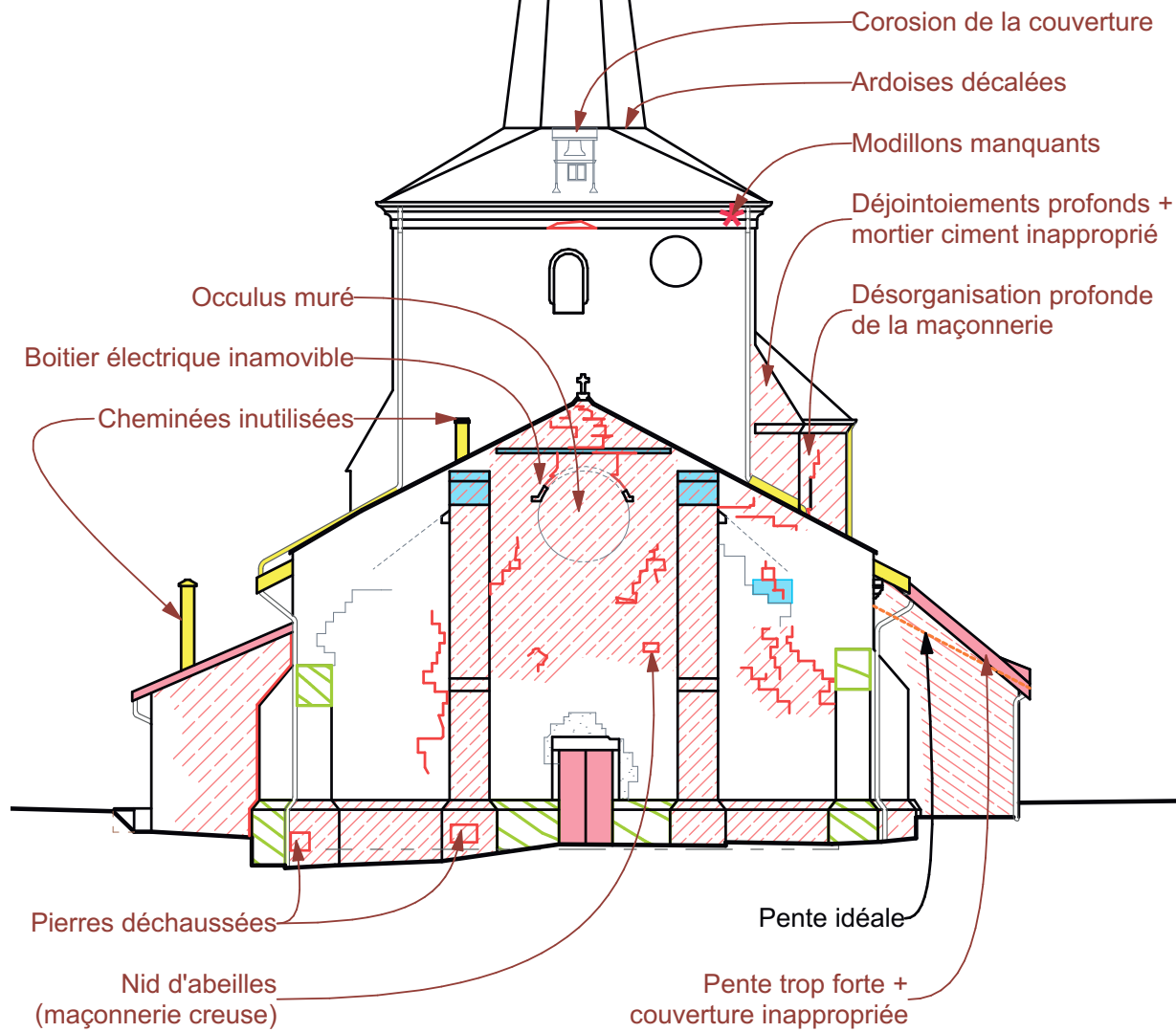
Élévation de la façade occidentale (diagnostic)
