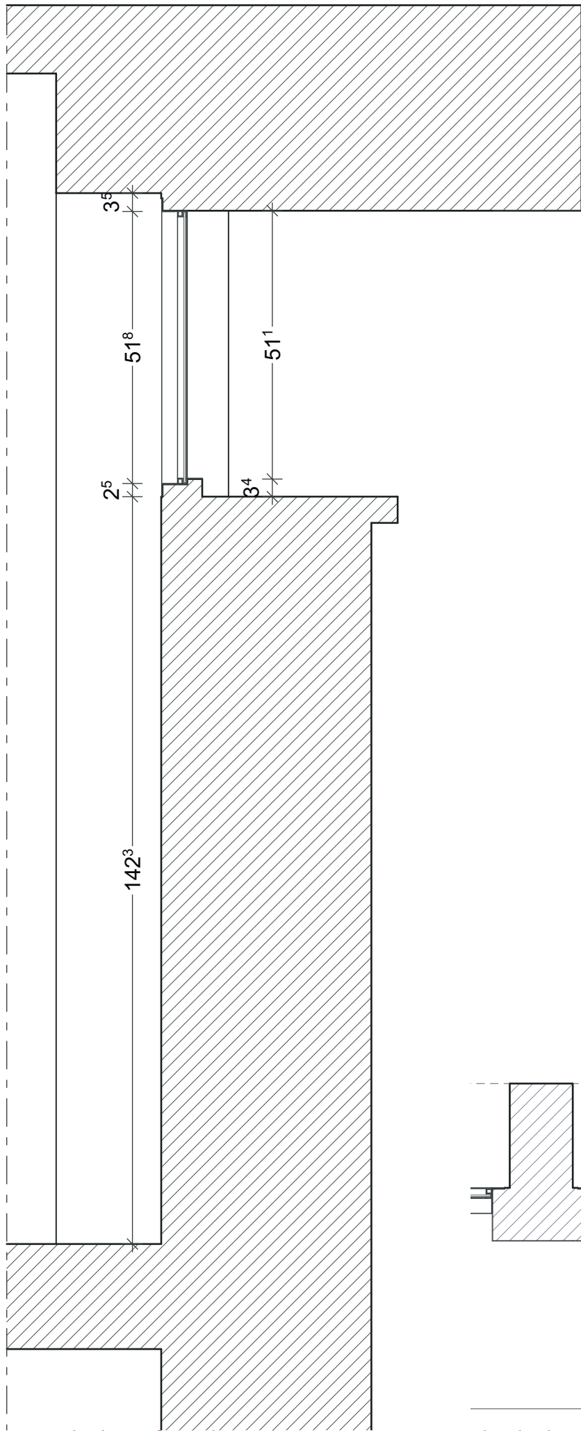
Coupe du châssis fixe (éch : 1/10)
