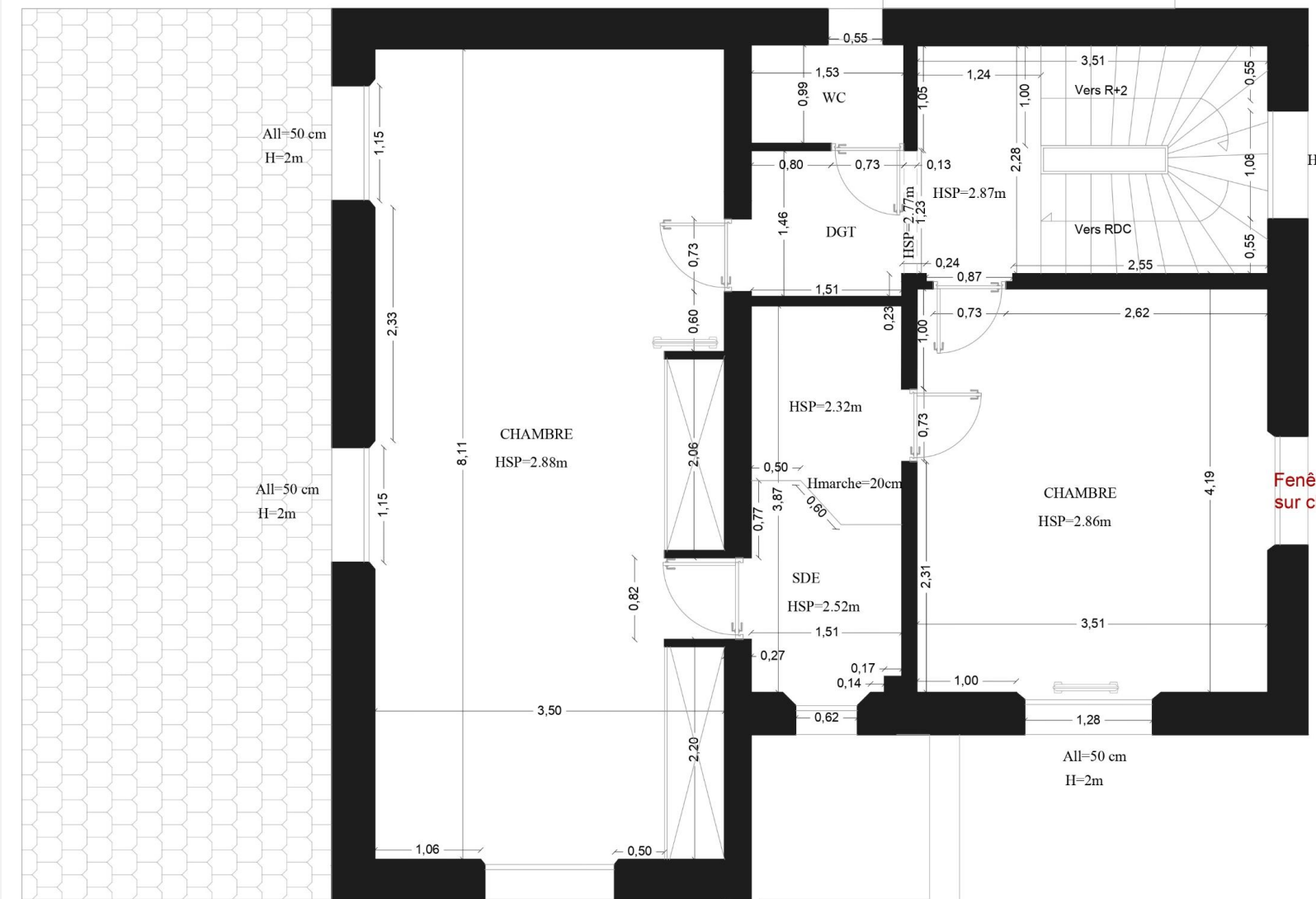
ETAGE- EXISTANT
