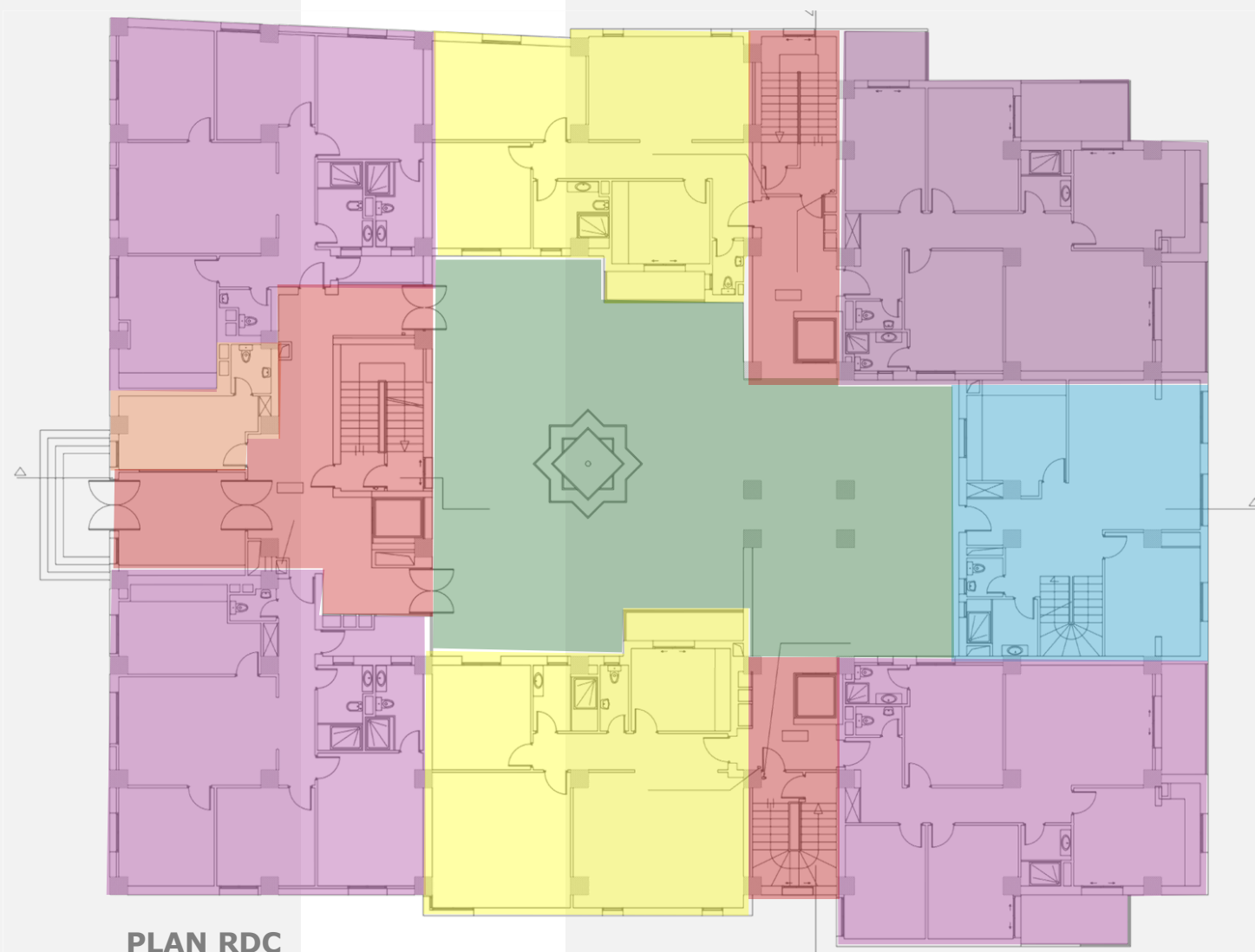
PLAN RDC
