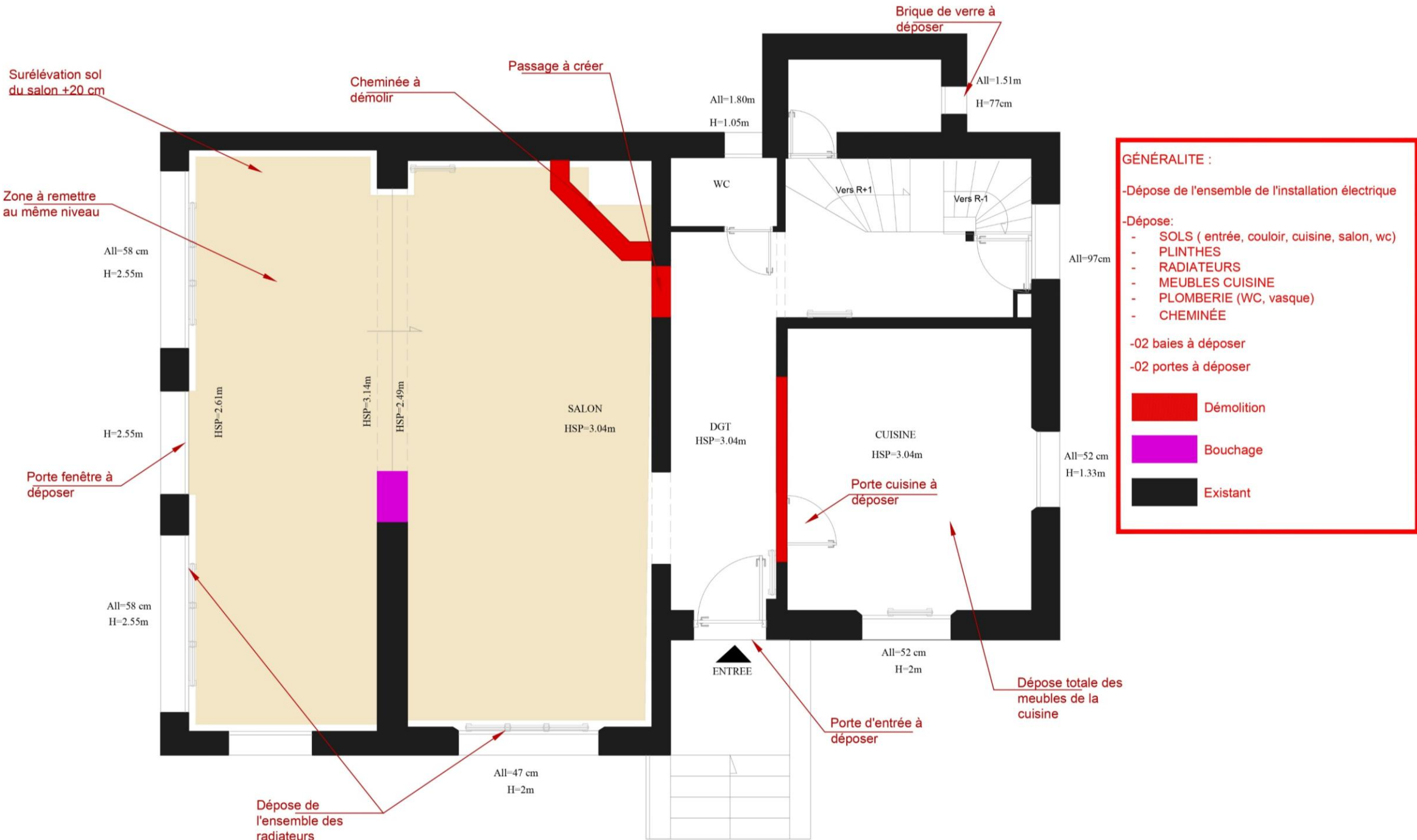
RDC-LOT DÉMOLITION
