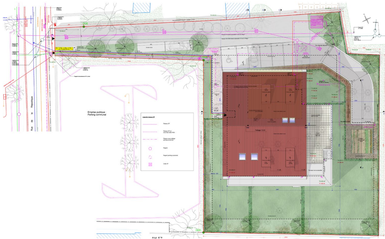
Plan Masse - 1.100
