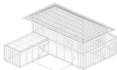
Axonométrie structure bois
