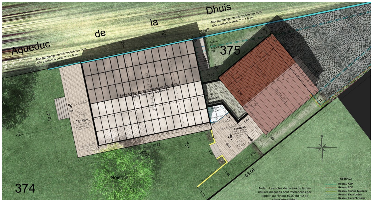
Plan Masse - 1.200
