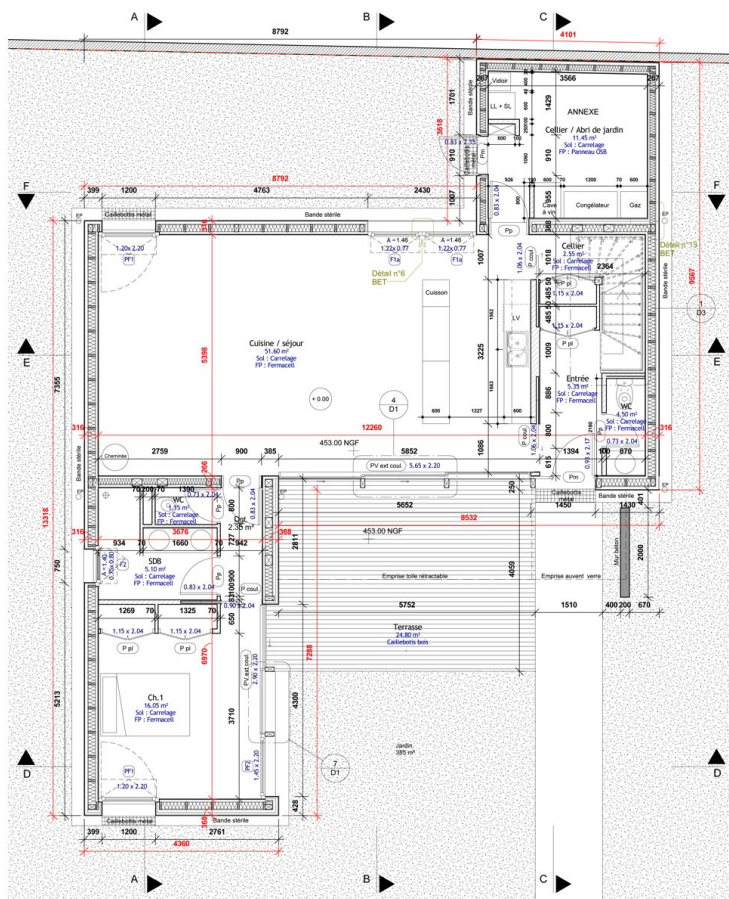
Plan RDC - 1.50
