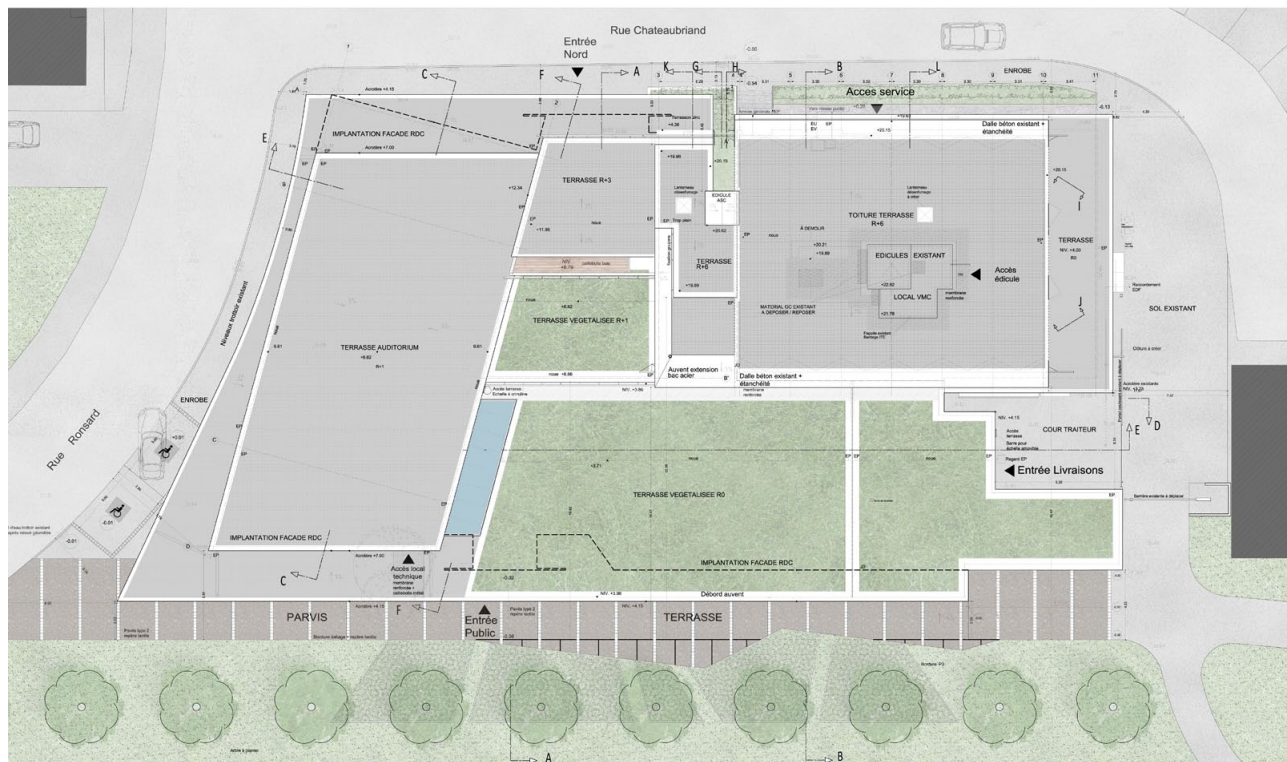
Plan Masse - 1.100
