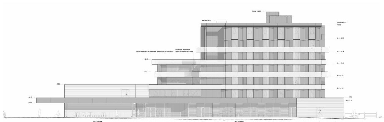
Façade Sud Est - 1.100
