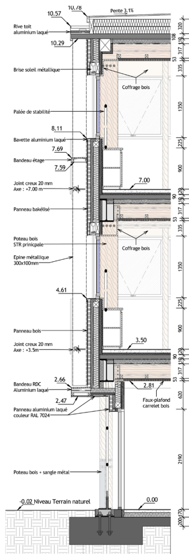
Coupe détail - 1.30
