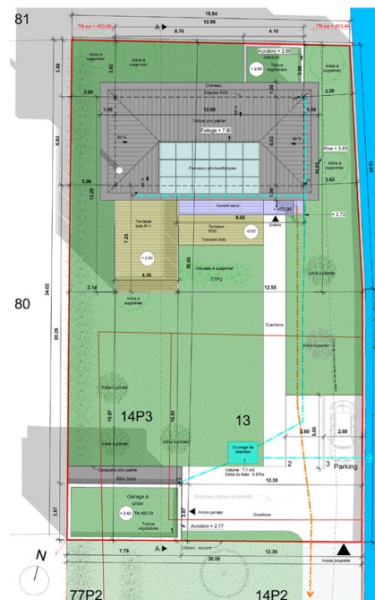
Plan masse - 1.100
