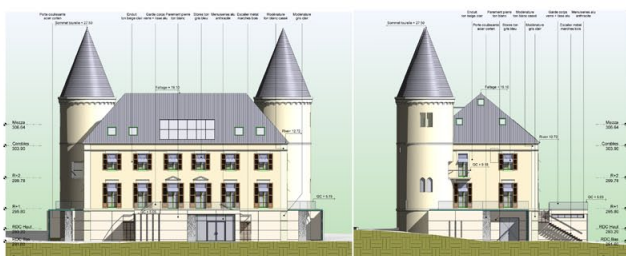
Façades - 1.200
