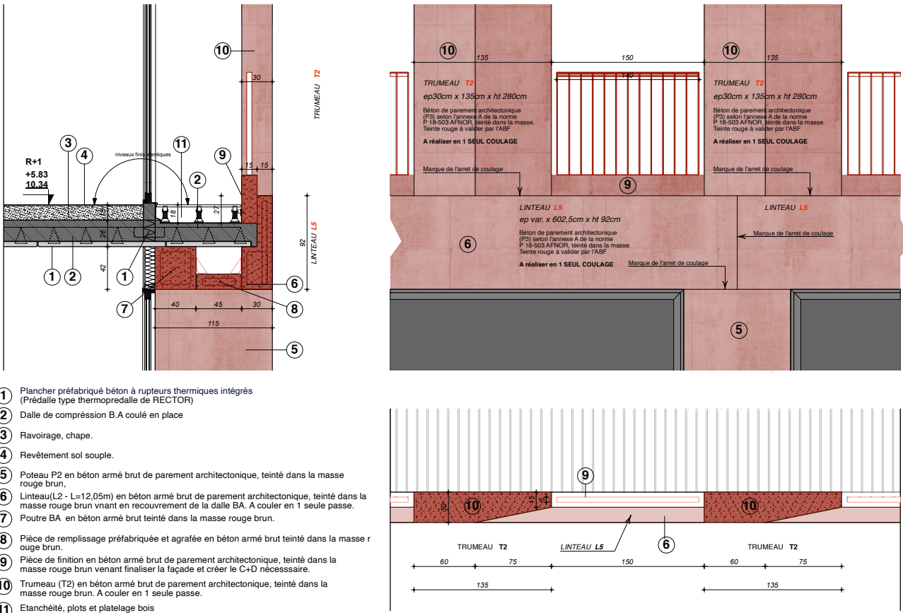
Détail de composition et calepinage des éléments béton teinté
